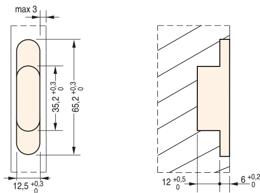
Misure della cava Slot measurement Mesures de l'encoche Abmessungen der Aushöhlung
