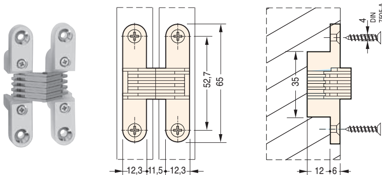
Misure della cava Slot measurement Mesures de l'encoche Abmessungen der Aushöhlung
