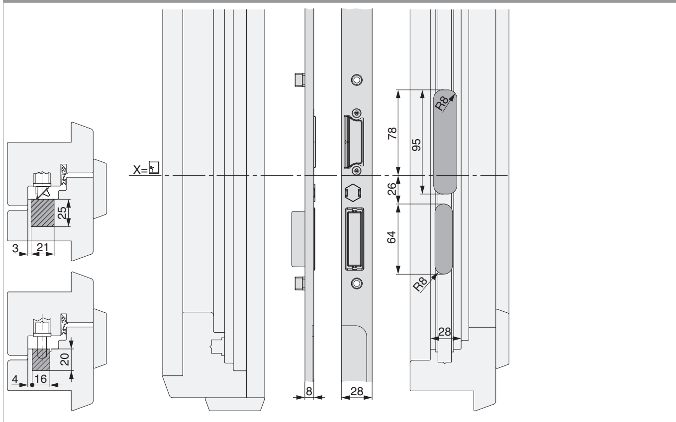
Dettaglio B
