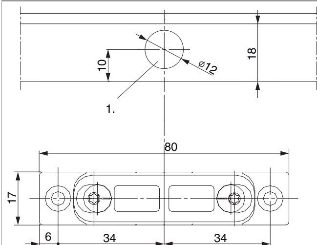
Scontri catenaccio con perni di posizionamento
