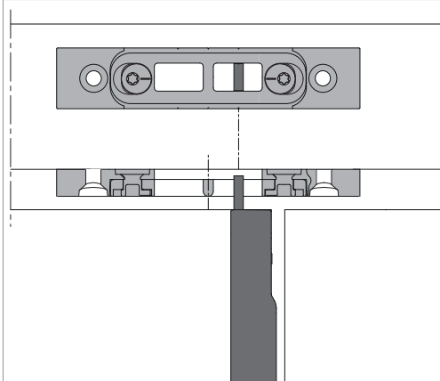
Finestra a 2 ante con 1 catenaccio
