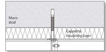
Modello / Model Supporto per cappotto per pioli spagnolette Stirrup for insulating layer for espagnolettes stops
