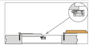
Modello / Model Fermo ad angolo avvitare Angled stop for screwing in
