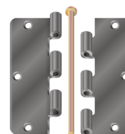
Serie / Series 140 Modello / Model Spina sfilabile decentrata Removable off-centre pin
