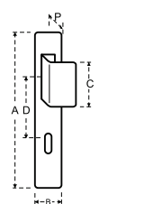
Maniglione reversibile con placca Reversible pull handle with backplate
